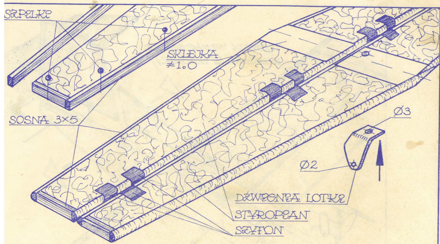
BUDOWA STATECZNIKA WYSOKOŚĆ, LOTKĘ, MONTAŻ ZAWIASÓW I DŹWĘGNE LOTKĘ
