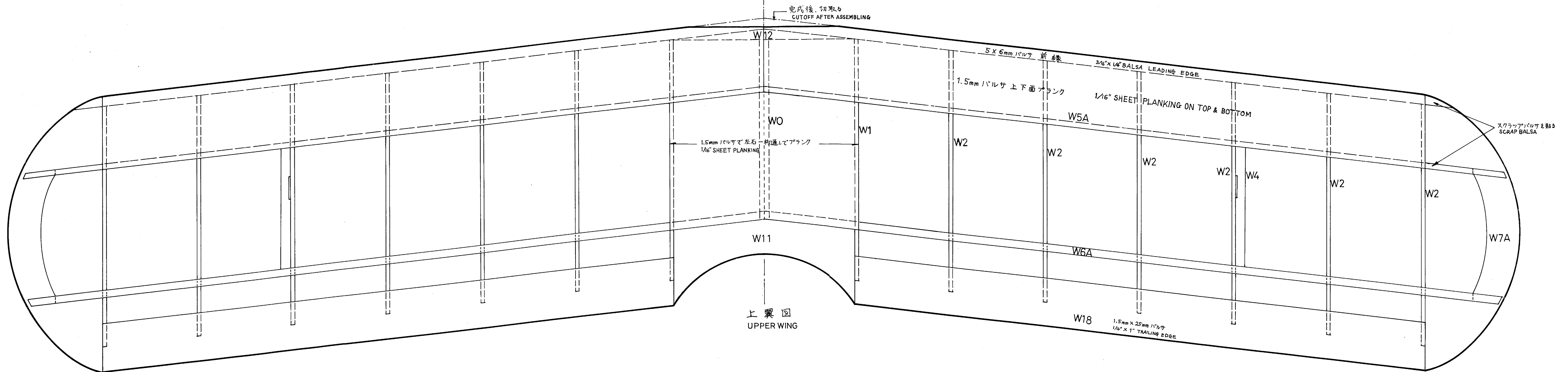
上翼組立図 UPPER WING
