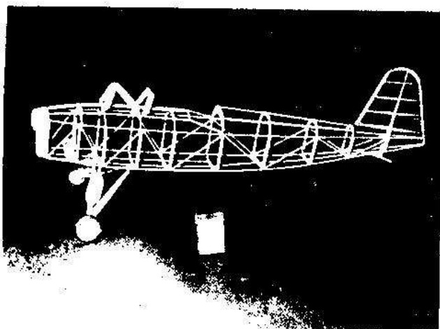
SZKIELET KADŁUBA
