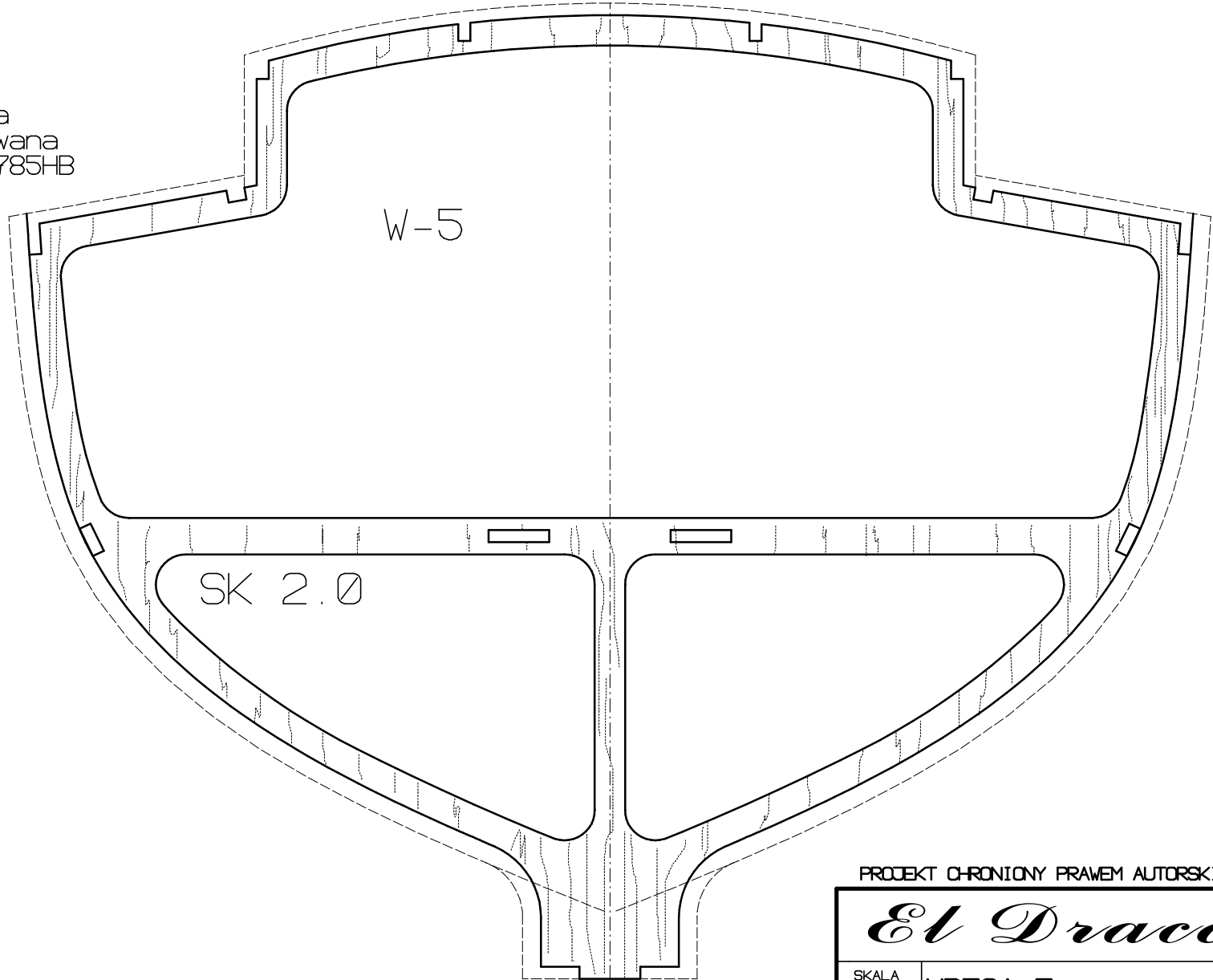
Półka na serwo windy
