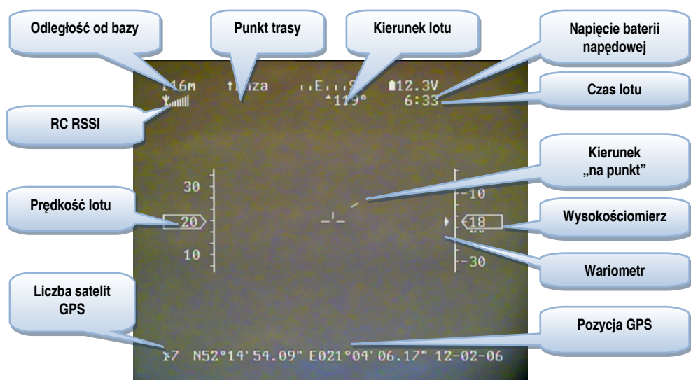
Ilustracja 2: Rozmieszczenie na ekranie i znaczenie informacji nawigacyjnych.
