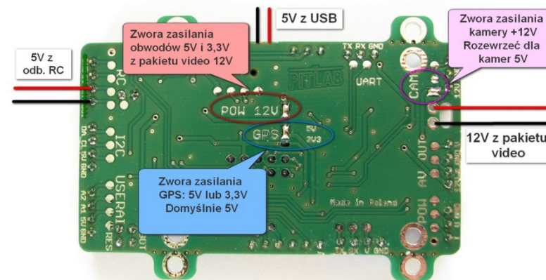
Ilustracja 3: Układ zwerek konfigurujących zasilanie OSD.
