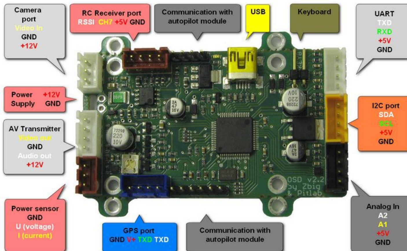
Ilustracja 4: Złącza OSD.
